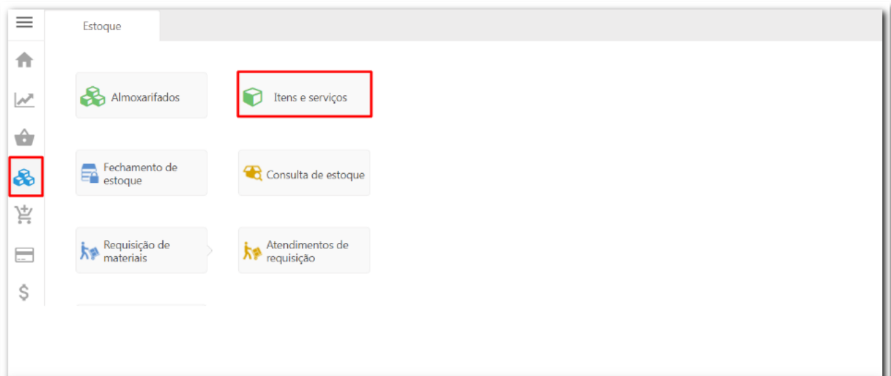
Figura 3 - Módulo Estoque
