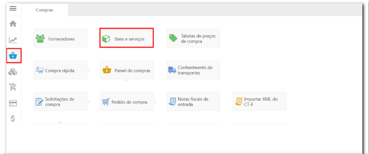
Figura 2 - Módulo Compras
