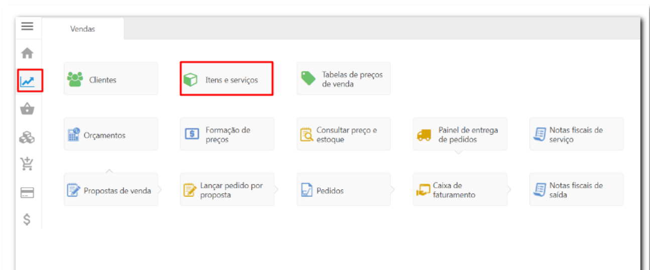
Figura 1 - Módulo Vendas
